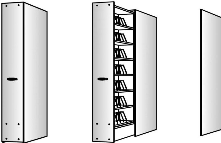
P211 HEIGHT 94” DEPTH 44” WIDTH 16”, 19”
